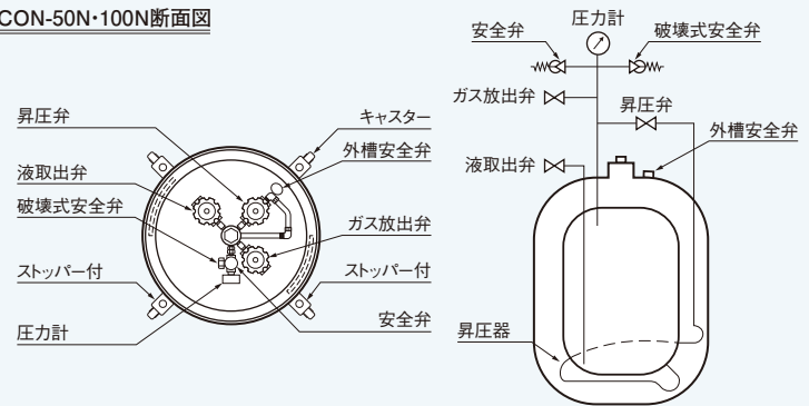
LICON-50N・100N断面図
